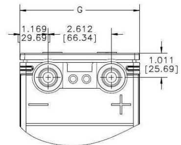
TEL 12-200 TFA
